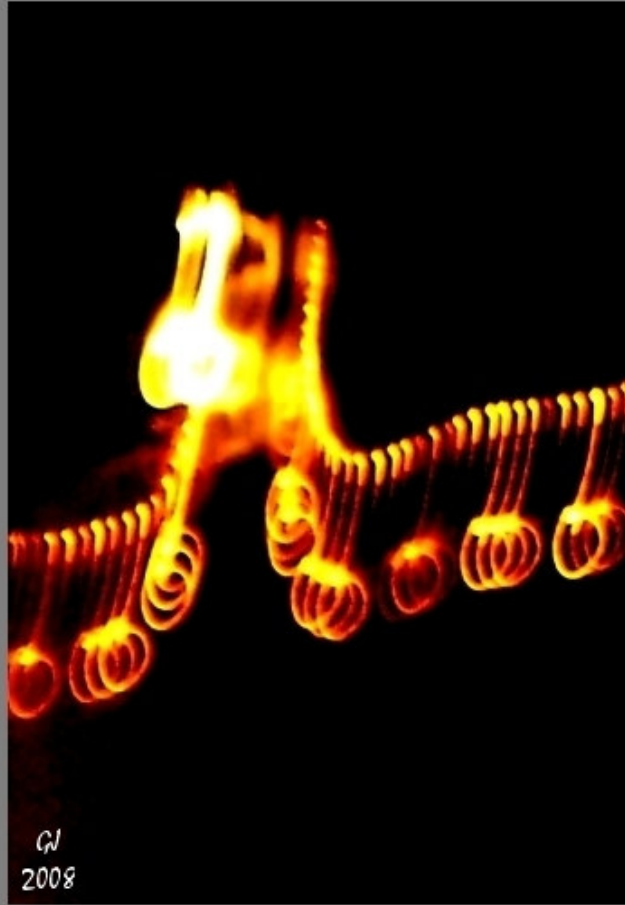
neutrino flavors
